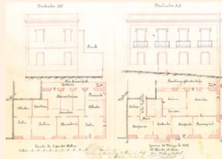
Plànol del permís d'obres de la rectoria vella aprovat el 27 de desembre de 1891. Com podem veure, només es planificava construir planta baixa més pis i al final es construïren dues plantes. Font: AMCM.
