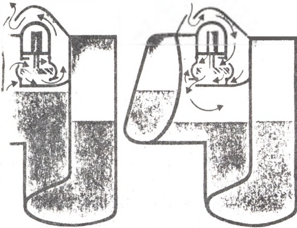
COLUMNA DE OSCILACIÓN DE AGUA
