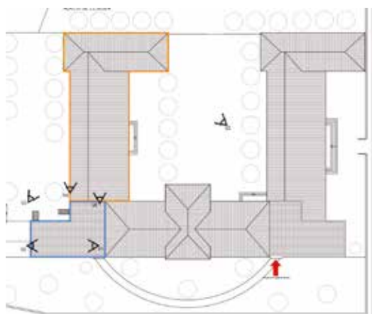
Plànol i Vista de la part de l'edifici on es farà l'actuació
