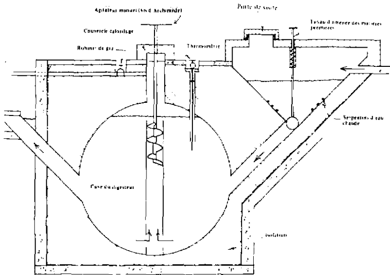
CRUQUIS D'UN DIGESTEUR SPHERIQUE AVEC DELANTALLET PRIMAIRES. LES MATIERES SONT RECUEILLIES des matières par une vis d'Archimede - Bassin de decantation et de culture d'algues
