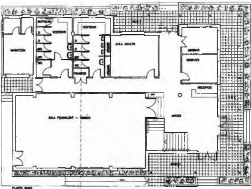
Planta baixa
