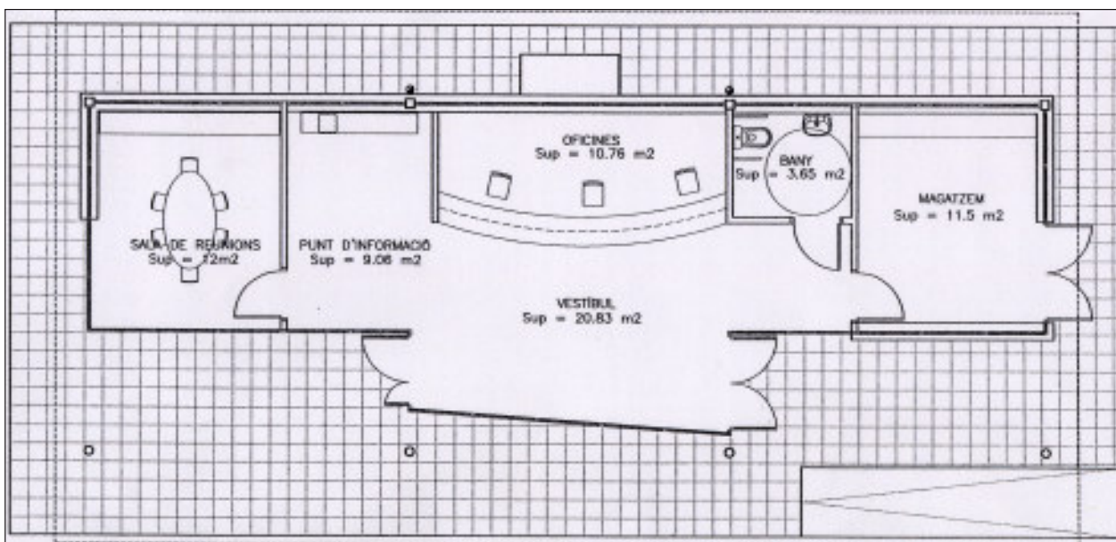
Plànol de la planta de l'edifici
