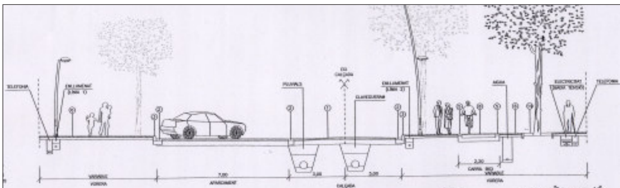
Tall d'un tram de l'Avinguda Doctor Furest
