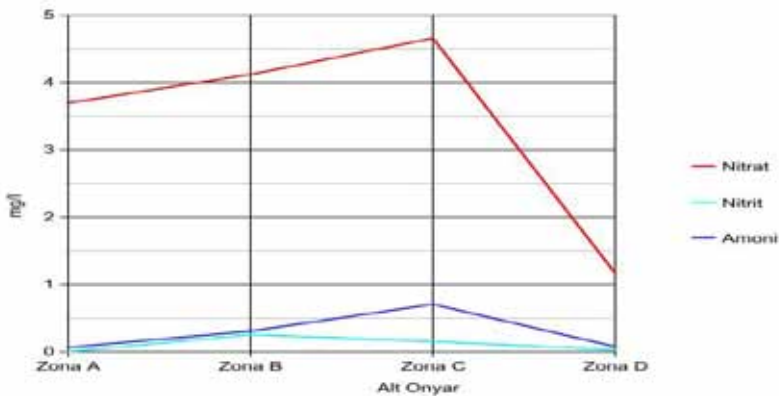
Evolució dels compostos nitrogenats al llarg de tota l'àrea de mostreig. Font: Menció, A & Mas-Pla, J 2004.
