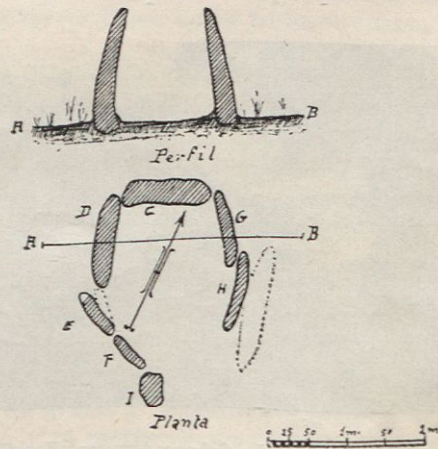
Fig. 135. — Planta i secció del sepulcre dels Arreganyats
