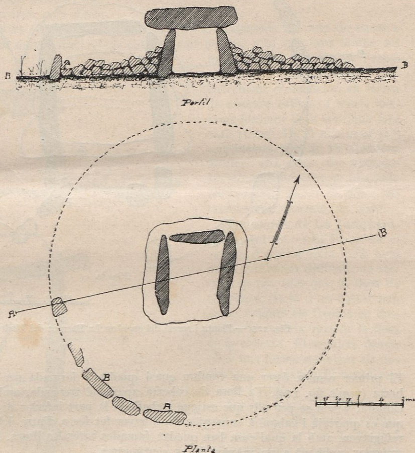
Fig. 124. — Planta i secció del sepulcre La Llosa de la Jassa d'En Torrent (L'Estrada)
