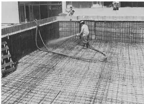
Vista de dues fases de la construcció de la piscina municipal.
