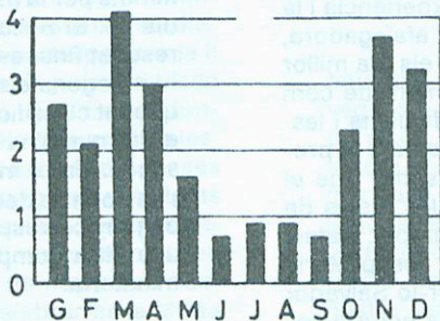
Gràfic n.º 3 Nombre de vegades en que entra Tramuntana segons el mes de l'any.
