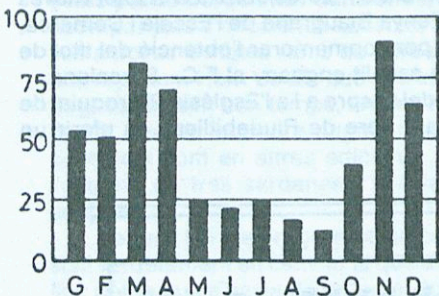
Gràfic n.º 2 Nombre d'hores de Tramuntana segons els mesos de l'any.
