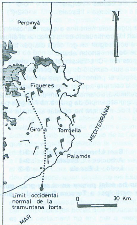
Gràfic n.º 1 Direcció i força del vent durant un dia típic de Tramuntana. (Observacions del 25 de novembre de 1977).
