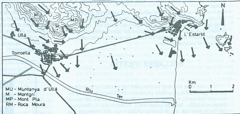
Gràfic n.º 4 La modificació de la direcció del vent és especialment important a la vessant sud de les muntanyes.
